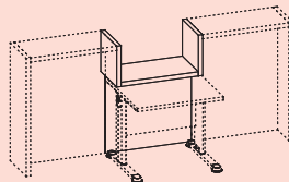
REBH080 80x40x73
